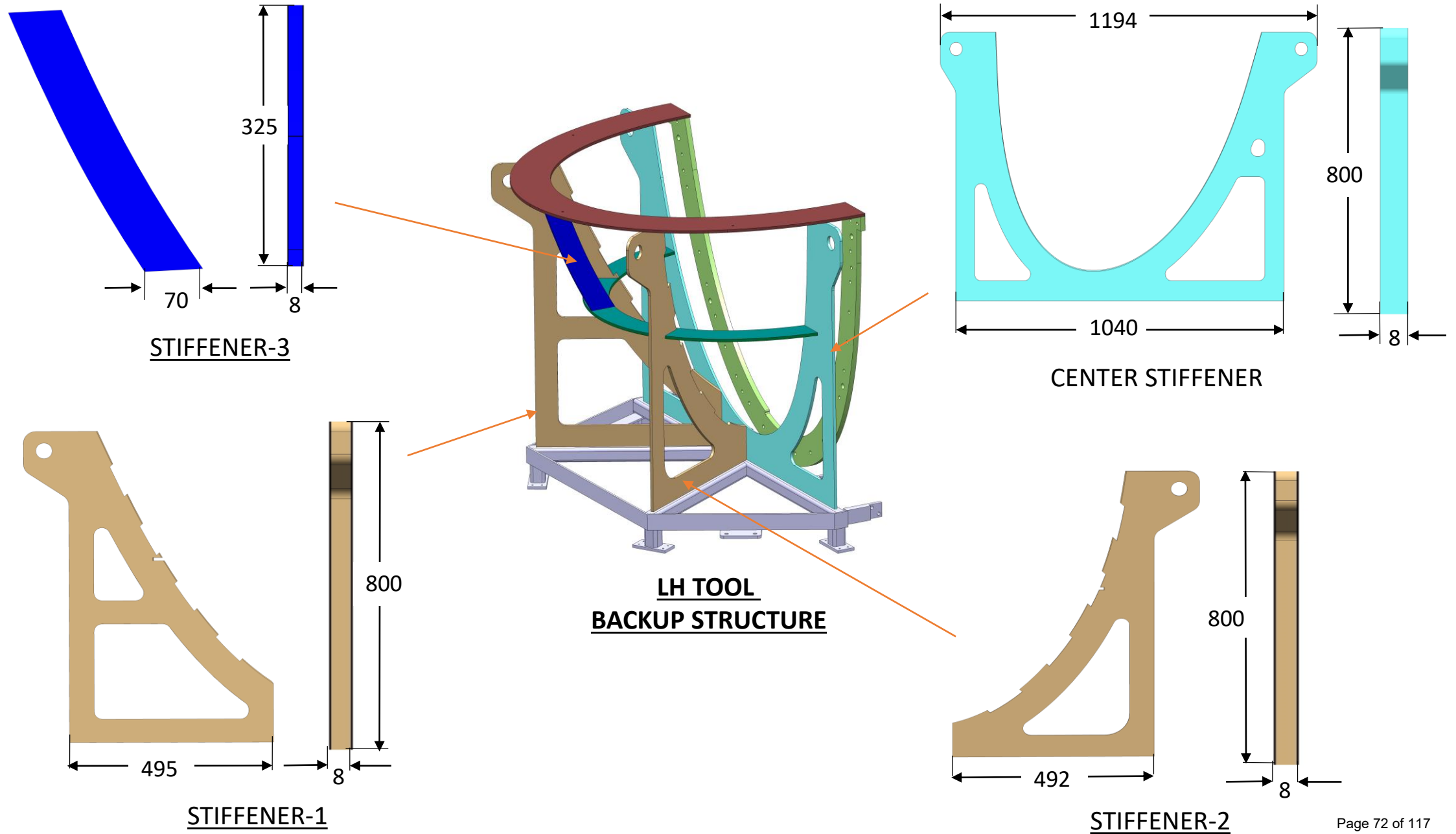
Fig. 06. LH TOOL STIFFENER DETAILS
