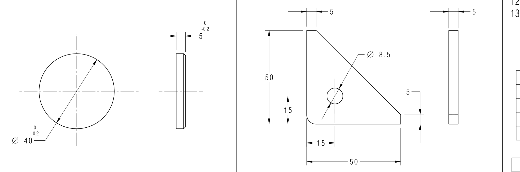
DETAIL OF ITEM NO:3 SCALE:1:1
