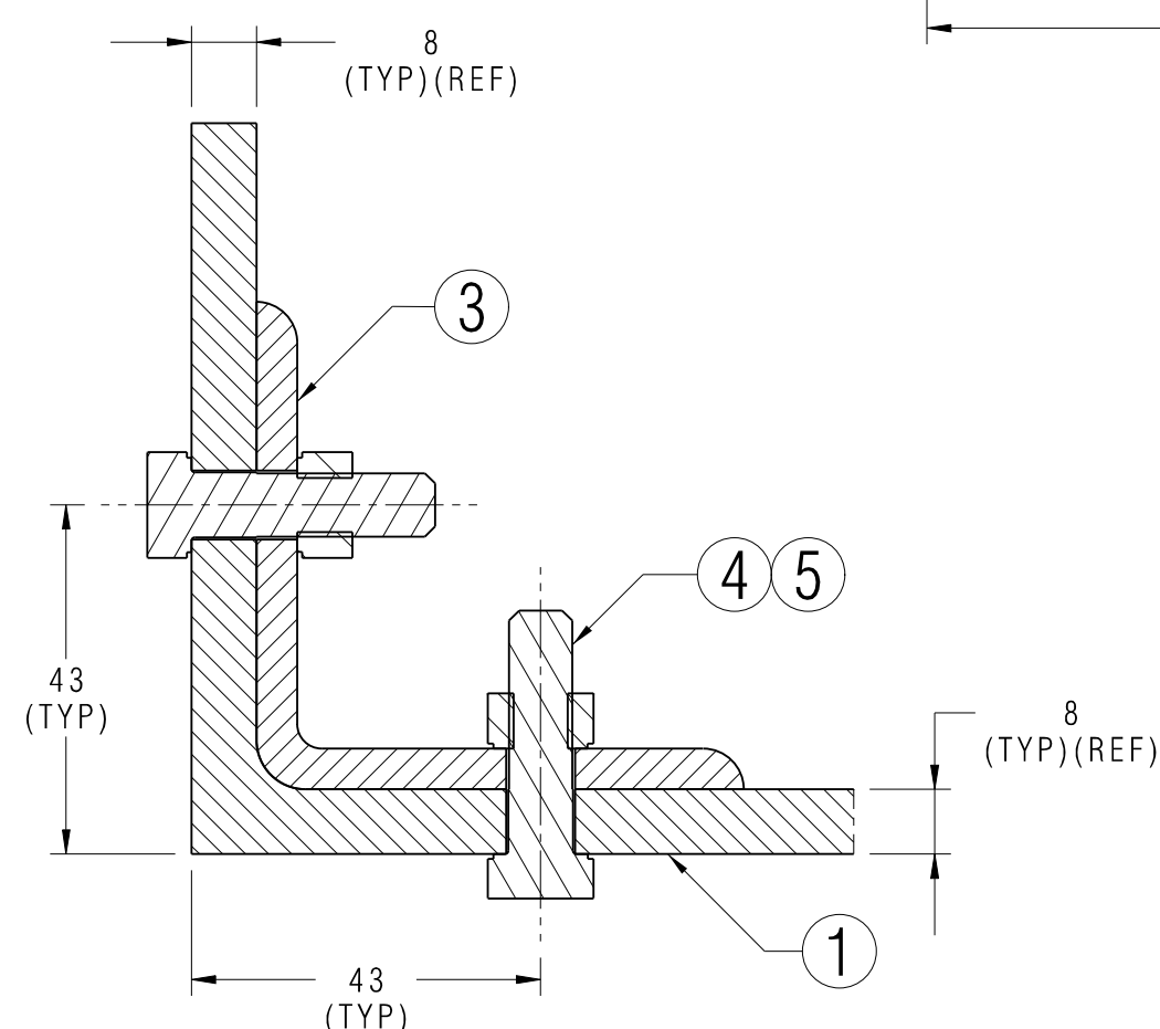
SECTION-DD SCALE: 2:5
